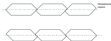
Схема подачи пластин магнитопровода
