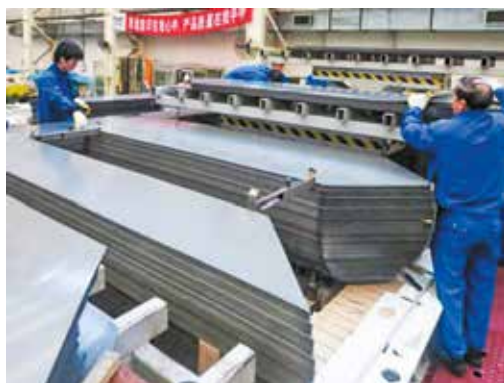
Сборка магнитопровода
